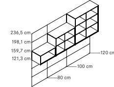
Rehausses à portes à battant, 1 à 3 haut. classeur
