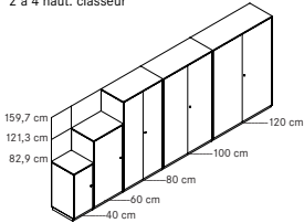
Armoire à portes à battant, 2 à 4 haut. classeur
