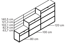
Armoire combinée tiroir/dossier suspendu, 1,5 à 3,5 haut. classeur
