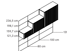
Rehausses à portes coulissantes, 1 à 3 haut. classeur
