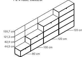
Armoires à dossier suspendu, 1 à 4 haut. classeur
