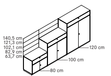
Armoire combinée tiroir/dossier suspendu, 1,5 à 3,5 haut. classeur
